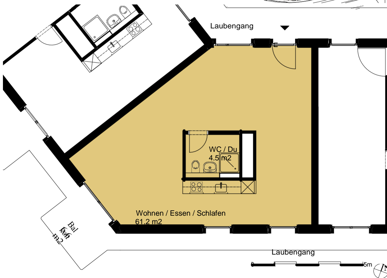
Grundriss 1:100
